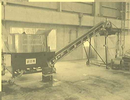
袋詰め機
